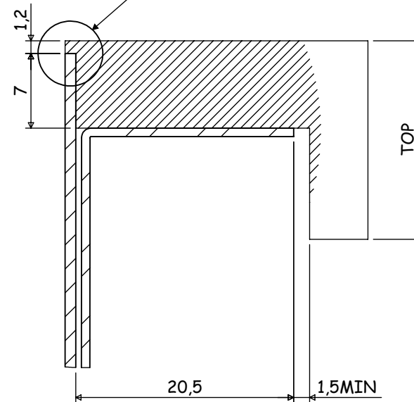
SORMONTO BORDO VASCA
