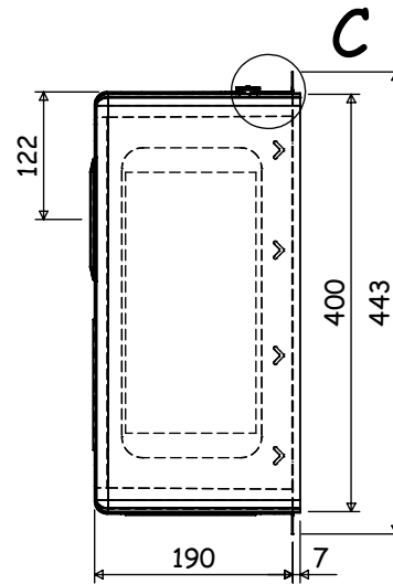
SEZIONE A-A
