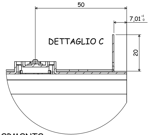
SORMONTO BORDO VASCA
